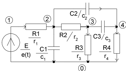
Рис. 1. Схема электрическая
