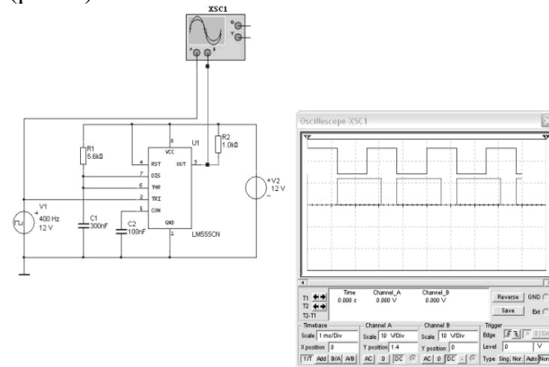
Рис. 1. Моделювання схем в Multisim
