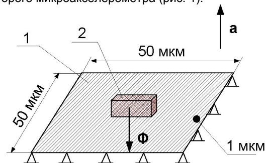
Рис. 1. Расчетная схема микроакселерометра.
